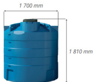
CUVE CEP 3 000
